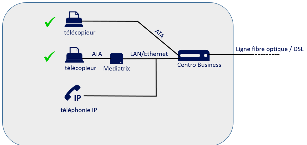
Illustr. 2: Smart Business Connect avec centraux téléphoniques virtuel (Trunk) et télécopieur analogique
