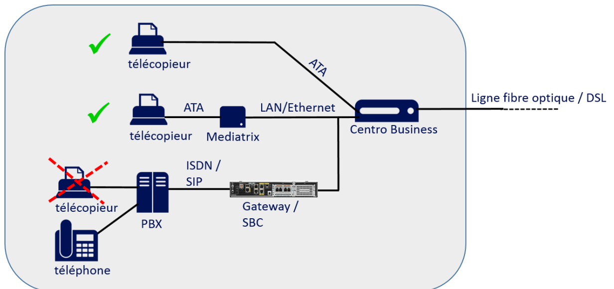
Illustr. 1: Smart Business Connect avec centraux téléphoniques sur site (Trunk) et télécopieur analogique
